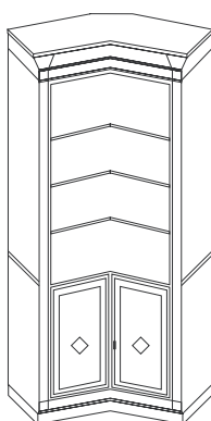
Art. 2075 Modulo Carlo X angolo 2 porte + giorno Carlo X corner module 2 open doors Modul Carlo X Eckelement 2-türig + offene Fächer L 86 P 46 H 232 m 3 1,95
