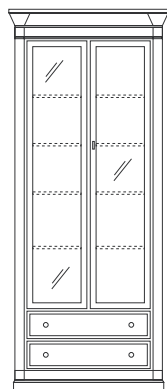
Art. 2086 Modulo Carlo X centrale 2 cass. + 2 porte vetro Carlo X central module 2 drawers + 2 glass doors Modul Carlo X Mittelelement 2 Schubladen + 2 Glastüren L 95 P 46 H 232 m³ 1,10
