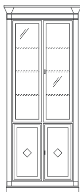
Art. 2071 Modulo Carlo X centrale 2 porte + 2 porte vetro Carlo X central module 2 doors + 2 glass doors Modul Carlo X Mittelelement, 2-türig + 2 Glas Türen L 95 P 46 H 232 m 3 1,10
