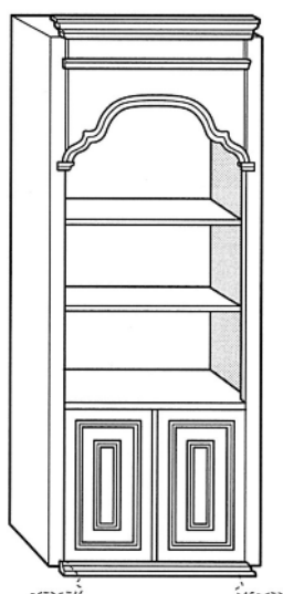
Art. 1515 Modulo Bizantino centrale 2 porte + giorno Central element 2 doors + open compartment Угловой Элемент 88x45x226 m³ 0,89
