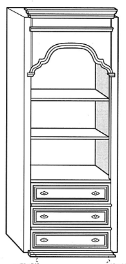
Art. 1517 Modulo Bizantino centrale 3 cass. + giorno Central element 3 drawers + open compart. Угловой Элемент 88x45x226 m³ 0,89
