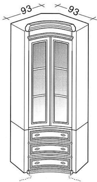
Art. 1510 Modulo Bizantino angolo 2 porte vetro Element 2 door corner piece Угловой Элемент 93x93x226 m³ 0,94
