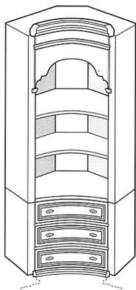
Art. 1511 Modulo Bizantino angolo a giorno Element open corner piece Угловой Элемент 93x93x226 m³ 0,94
